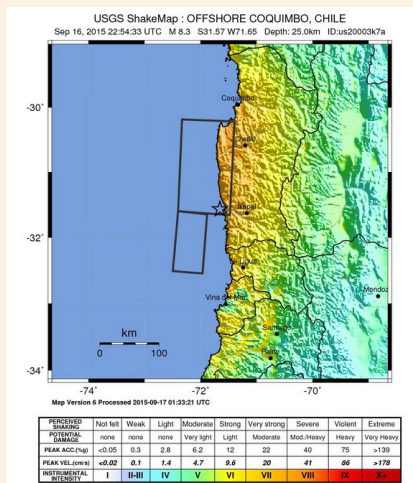
Fuerza del terremoto del 16 de septiembre 2015
